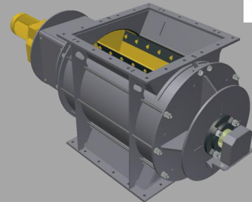
Zellenradschleuse Rotary valve
