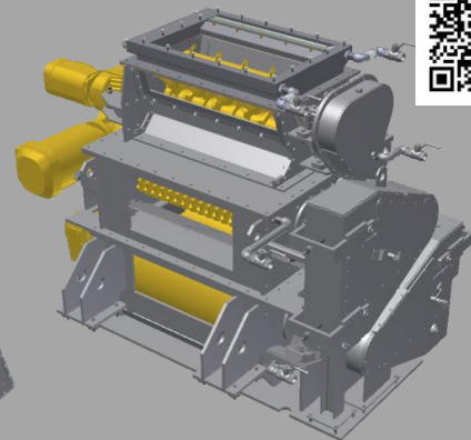
Walzenbrecher Roll crusher
