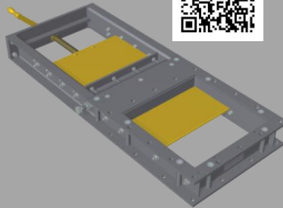
Schüttgutschieber Slide gate
